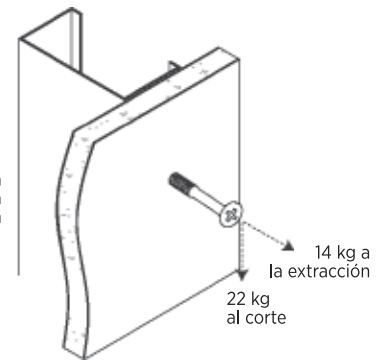
Carga Intermedia Tornillo S-1
