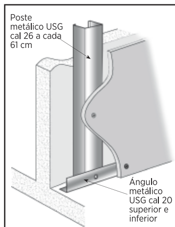
Lambrín a base de poste y ángulo
